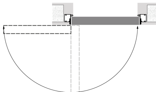
lewe, drzwi otwierane na zewnątrz
